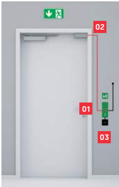
01 SafeRoute Basic-Set mit ST-VP Verteilerplatine 02 STV 1xx Türverriegelung 03 Bauseitige Zutrittskontrolle für Impuls-Ansteuerung der Entriegelung
