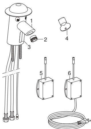
Figura 1: Rubinetteria per lavabo Bambini Geberit
