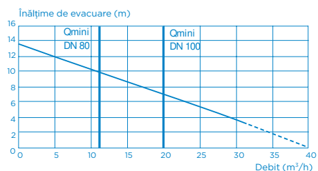
Cot evacuare SANICUBIC® 1 VX / SANICUBIC® 2 VX monofazic
