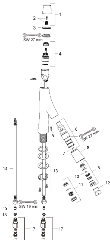
製品分解図
