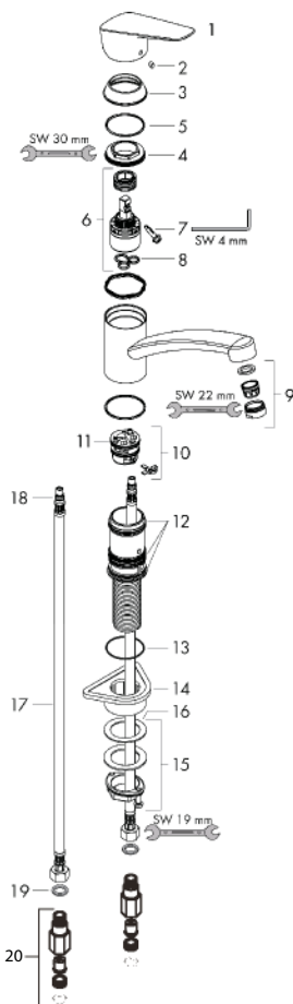
製品分解図
