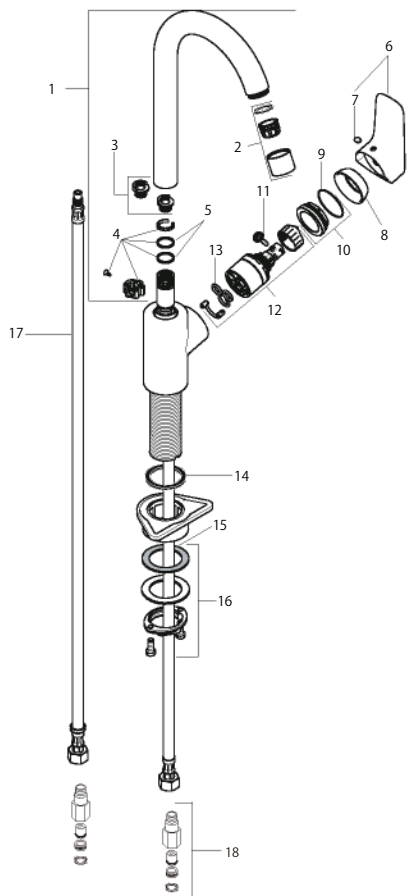
製品分解図
