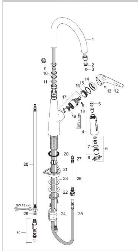
製品分解図
