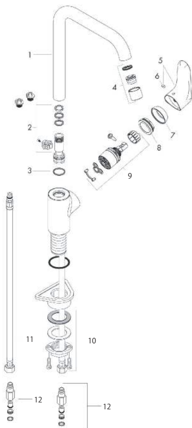
製品分解図
