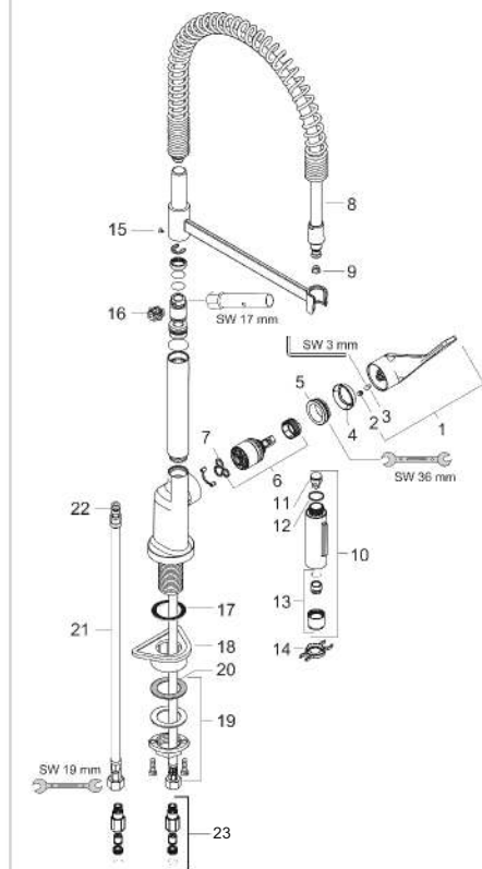
製品分解図
