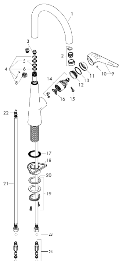
製品分解図
