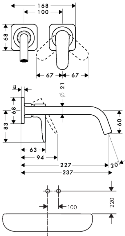
AXOR Citterio M 34116XXX
