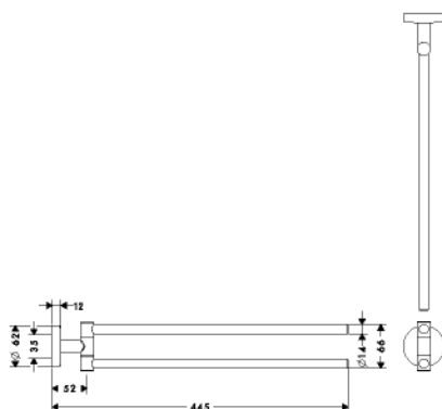
完成図
