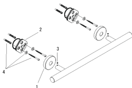
製品分解図
