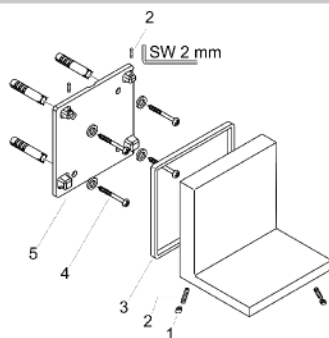
製品分解図
