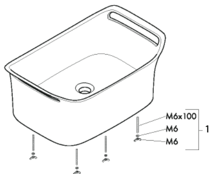
製品分解図
