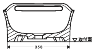
取付穴開口寸法
