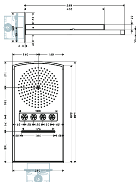
完成図
