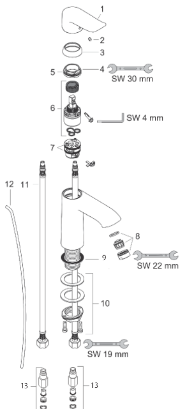
製品分解図
