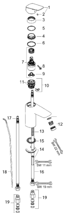
部品リスト
