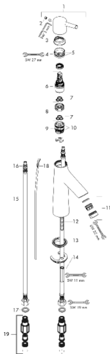
部品リスト
