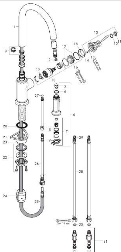
製品分解図
