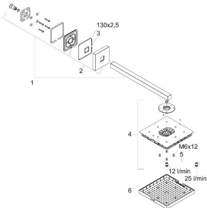
製品分解図
