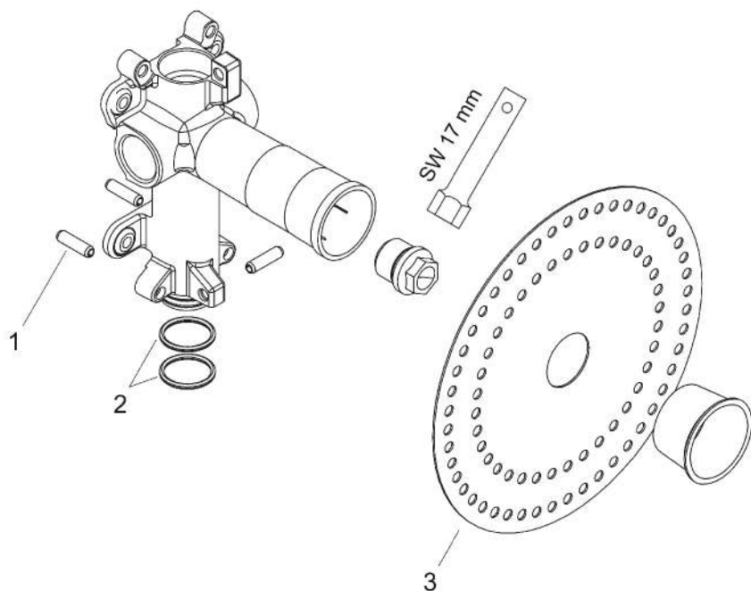
完成図
