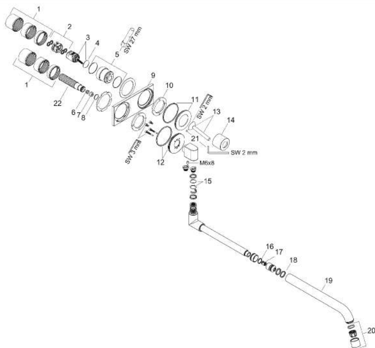
部品リスト
