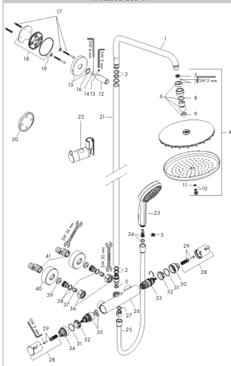
部品リスト
