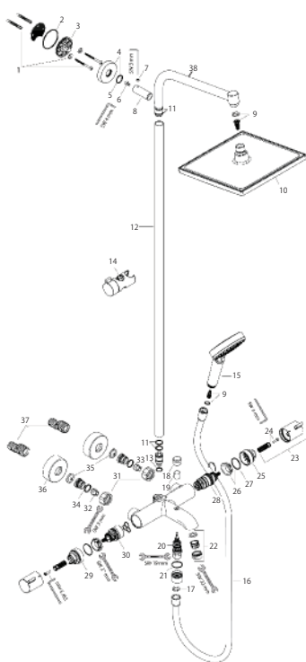
製品分解図
