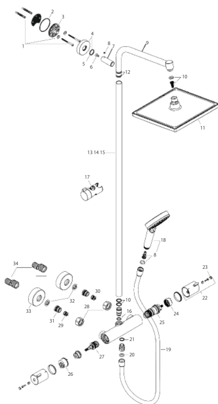
製品分解図
