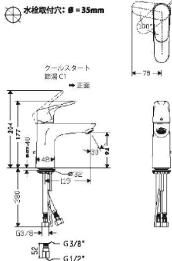
完成図
