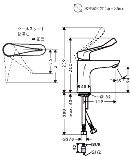
完成図
