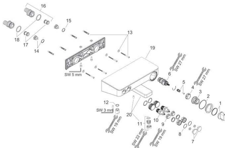
製品分解図
