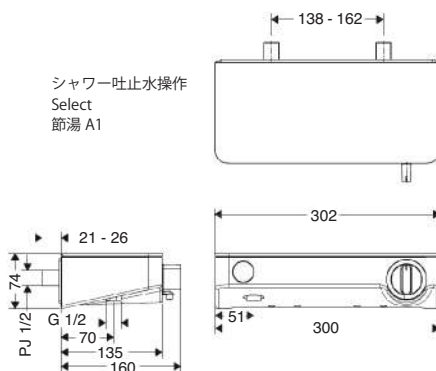
完成図
