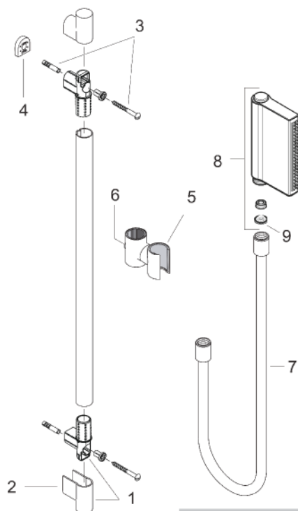
製品分解図
