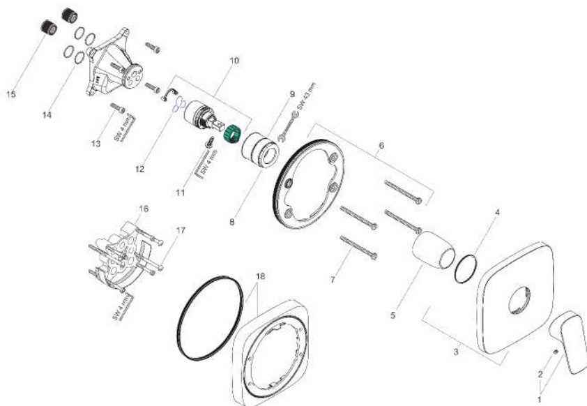
製品分解図
