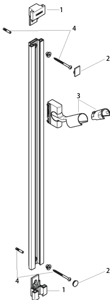
製品分解図
