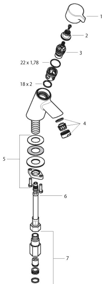
製品分解図
