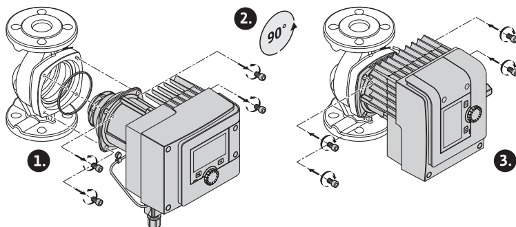
Fig. 8: Motor drehen
