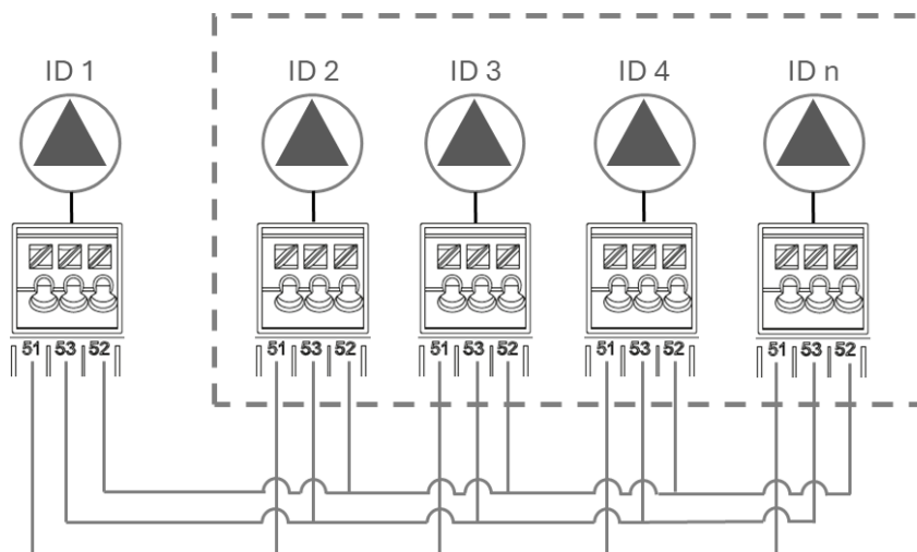
Fig. 46: Bus Wilo Net Verdrahtung
