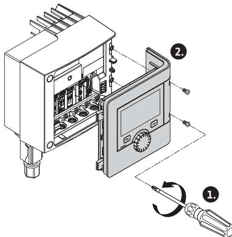
Fig. 92: Moduldeckel öffnen
