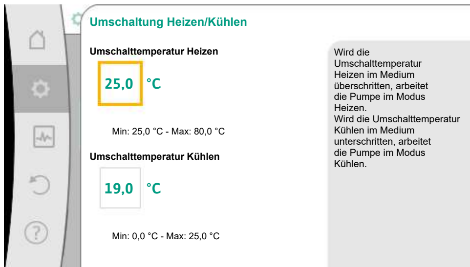
Fig. 43: Umschaltung Heizen/Kühlen_„Umschalttemperaturen“
