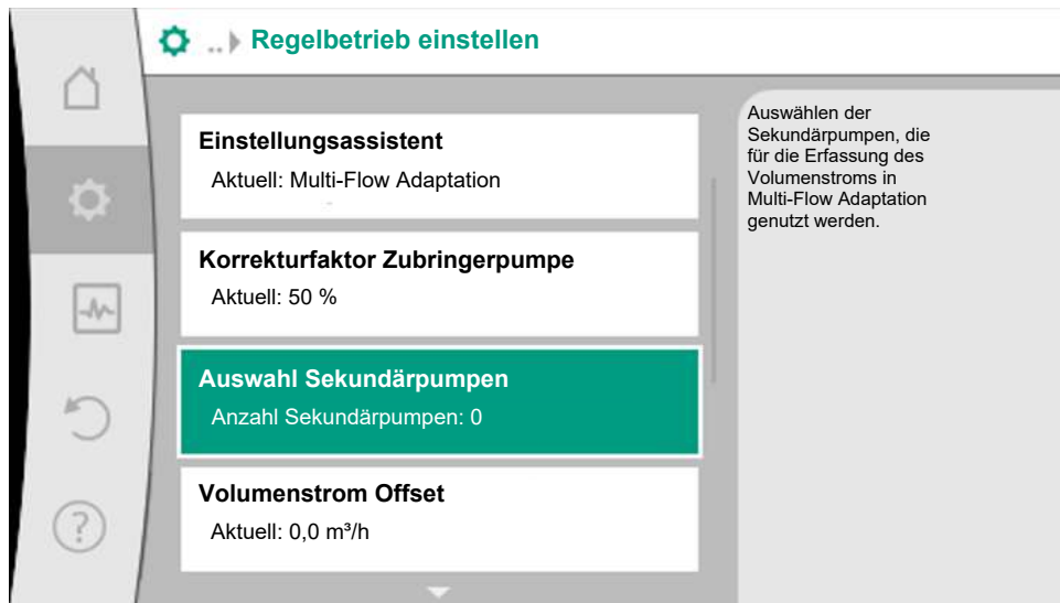
Fig. 51: Auswahl der Sekundärpumpen zu Multi-Flow Adaptation
