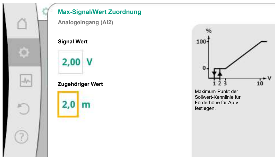
Fig. 76: Max-Signal/Wert Zuordnung
