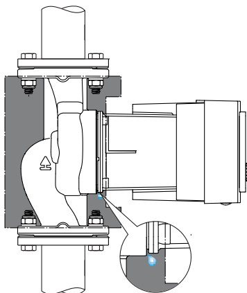
Fig. 9: Dämmen, Kondensatablauf freilassen
