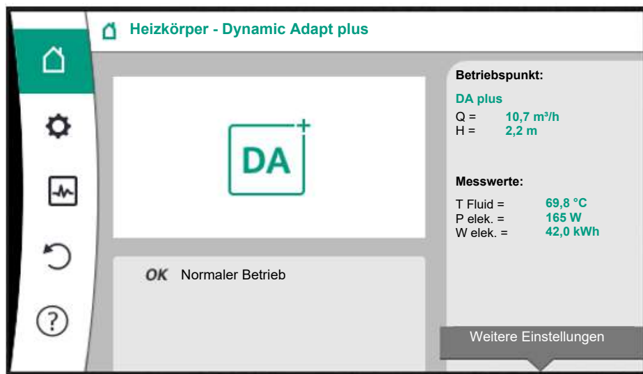
Fig. 19: Hauptmenü
