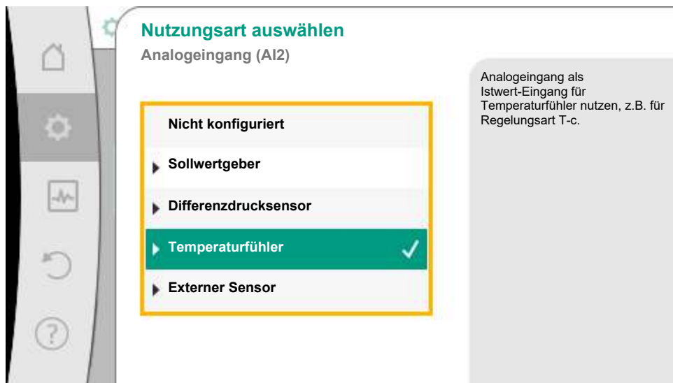
Fig. 78: Einstelldialog Istwertgeber
