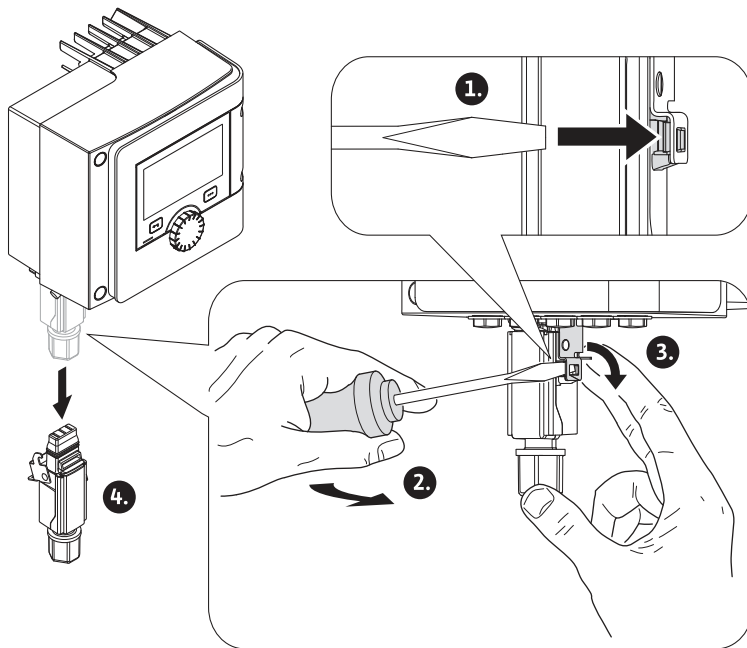
Fig. 91: Wilo-Connector demontieren
