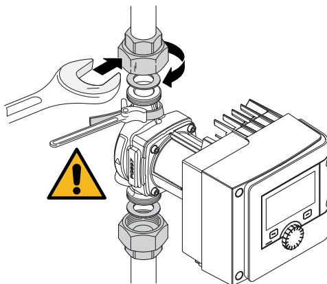
Fig. 7: Pumpe montieren
