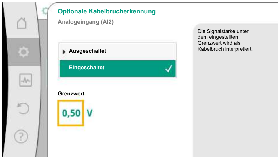
Fig. 72: Grenzwert Kabelbruch
