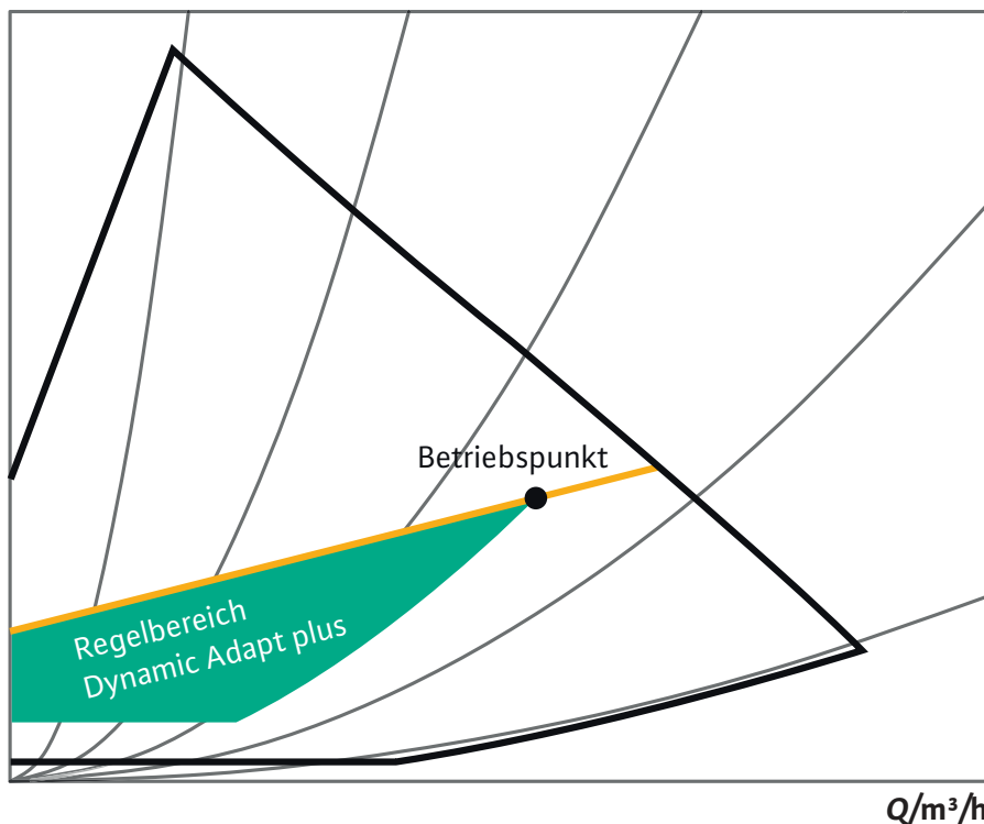
Fig. 28: Regelbereich Dynamic Adapt plus
