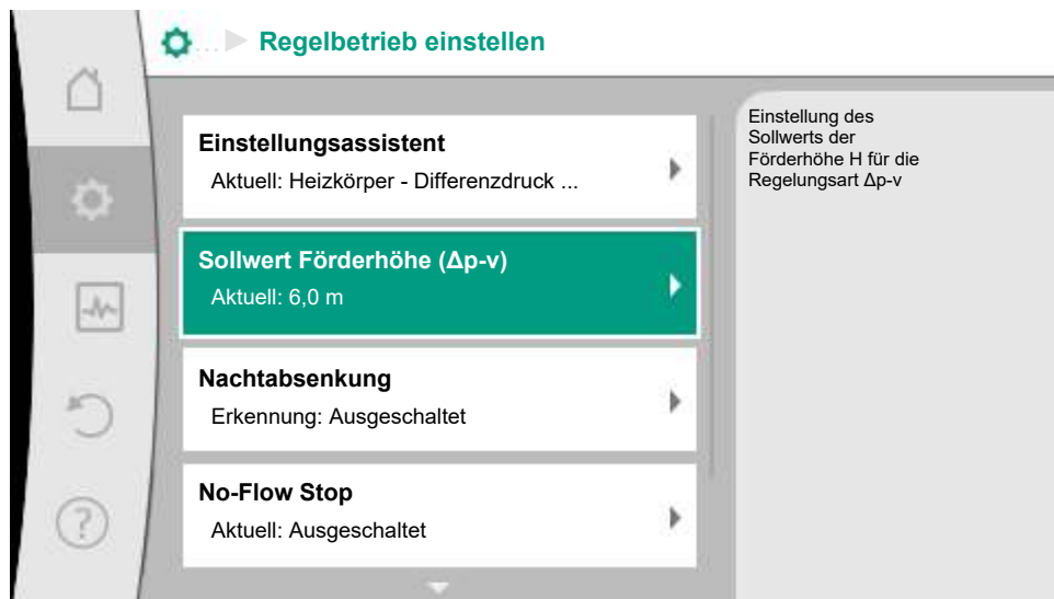
Fig. 64: Sollwerteditor
