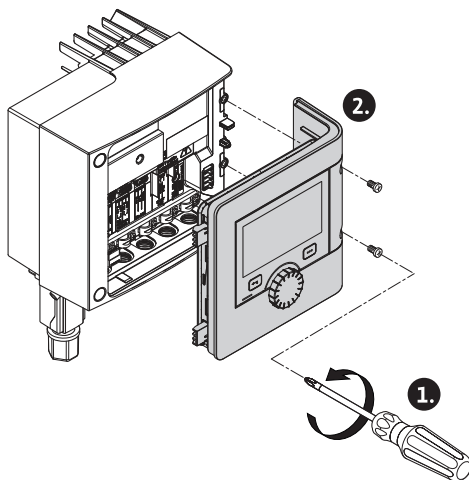
Fig. 13: Moduldeckel öffnen
