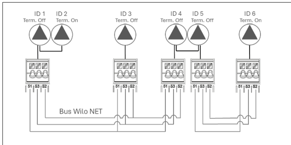
Fig. 47: Bus Wilo Net Adressierung
