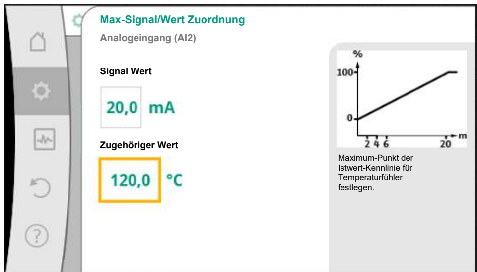
Fig. 81: Max-Signal/Wert Zuordnung Istwertgeber
