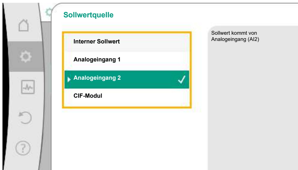
Fig. 67: Sollwertquelle
