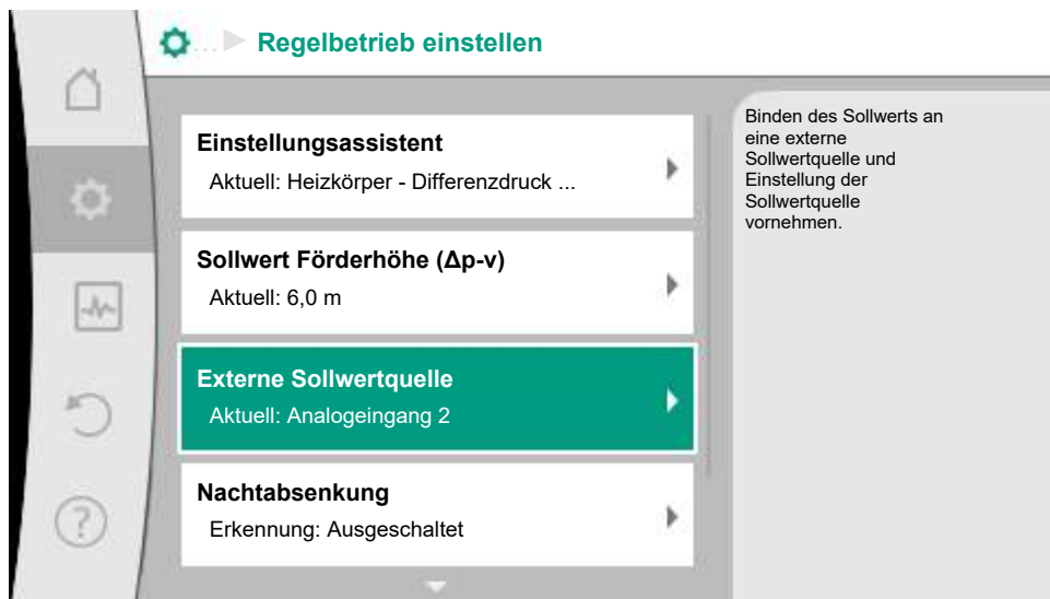
Fig. 66: Externe Sollwertquelle
