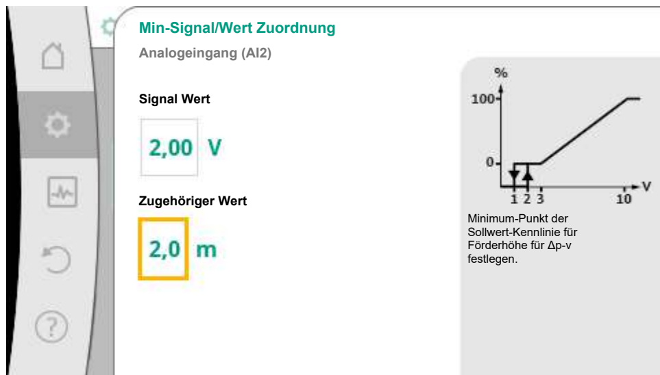
Fig. 75: Min-Signal/Wert Zuordnung
