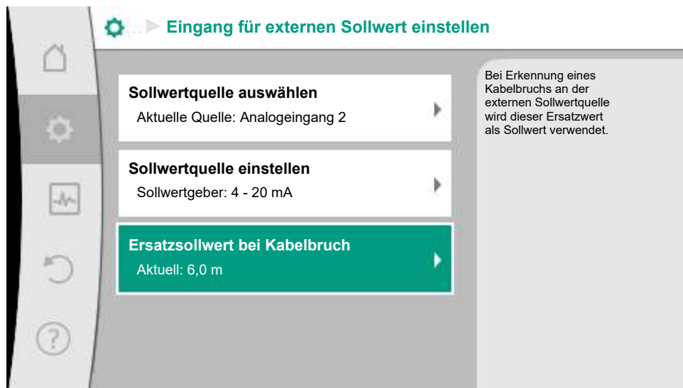
Fig. 77: Ersatzsollwert bei Kabelbruch
