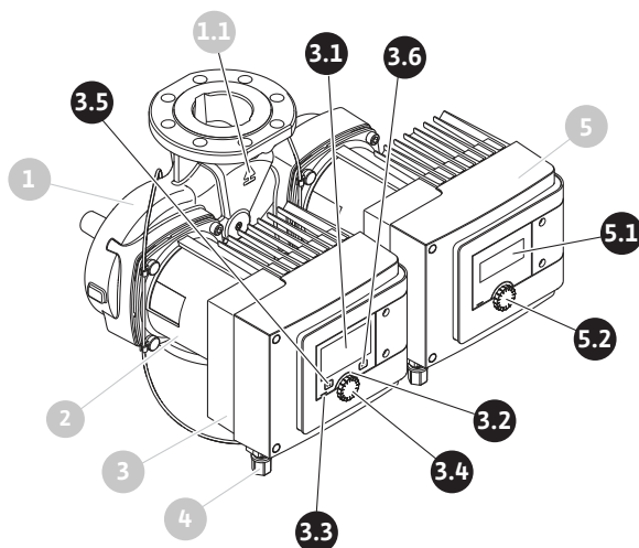
Fig. 17: Bedienelemente (Doppelpumpe)
