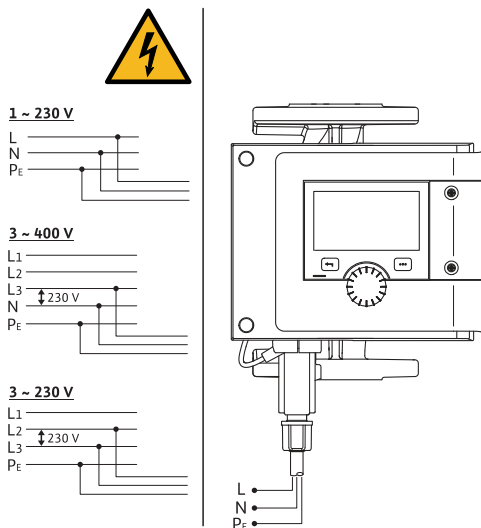
Fig. 11: Anschlussmöglichkeiten
