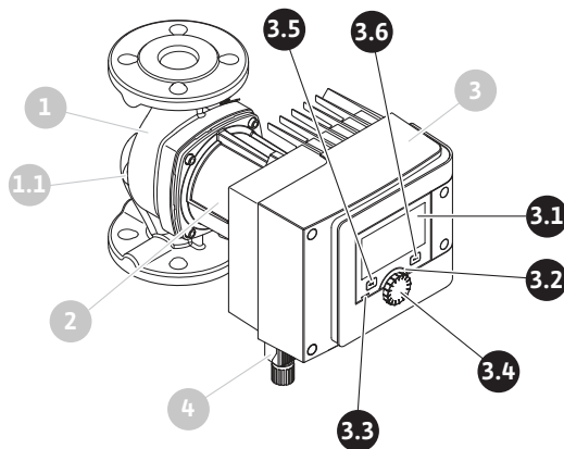
Fig. 16: Bedienelemente (Einzelpumpe)
