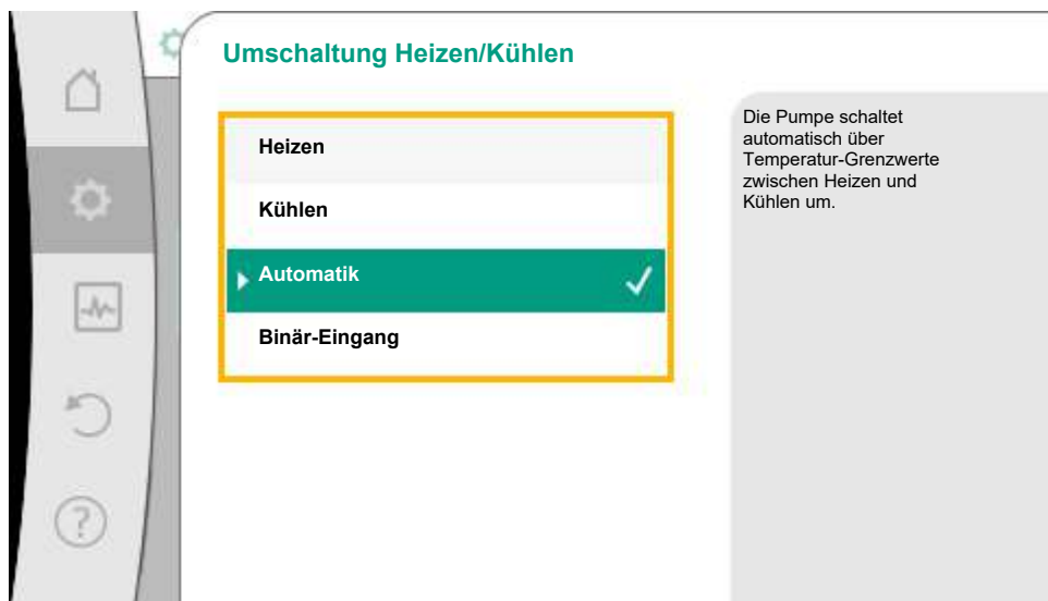
Fig. 42: Umschaltung Heizen/Kühlen_„Automatik“
