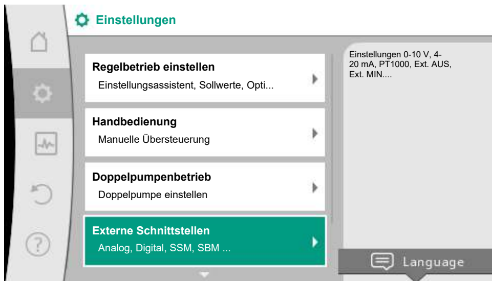
Fig. 48: Externe Schnittstellen
