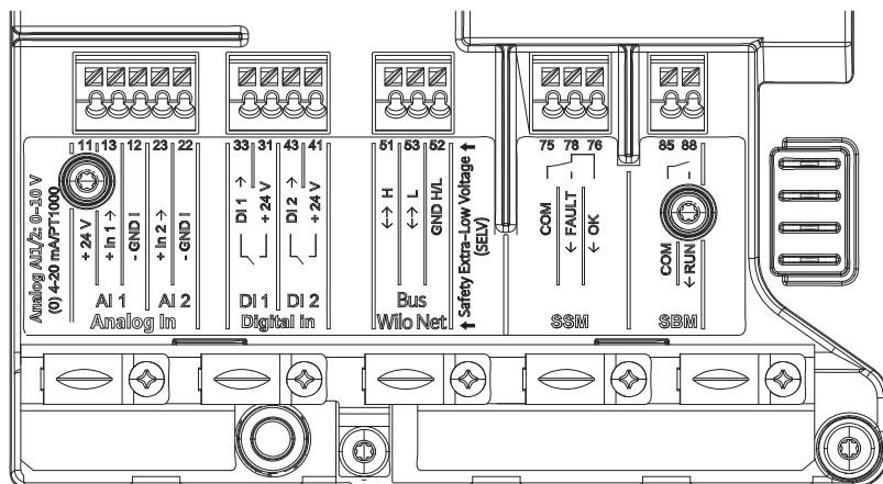
Fig. 14: Kommunikationsschnittstellen
