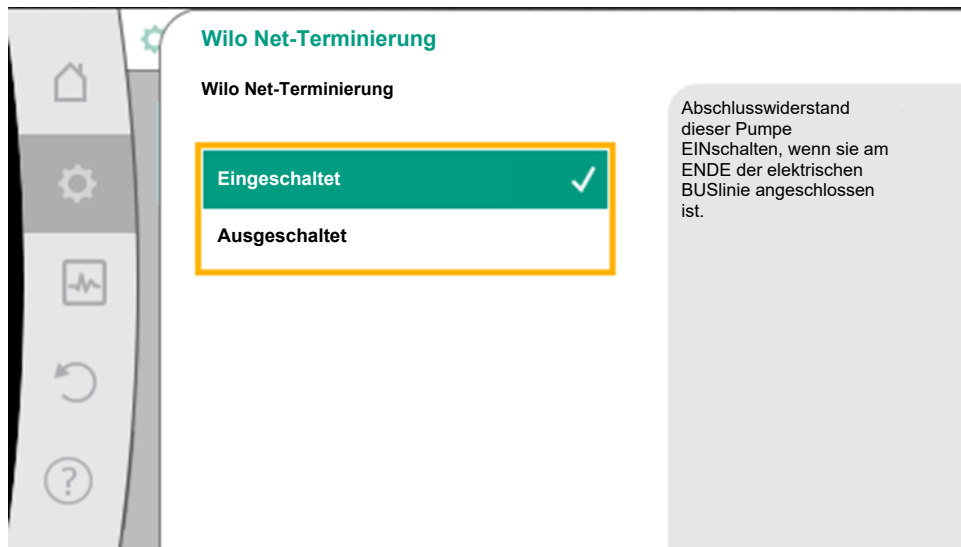
Fig. 50: Wilo Net-Terminierung
