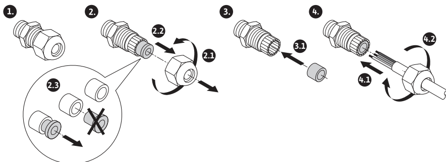
Fig. 10: Kabelverschraubung Ø 5 ... 10 mm
