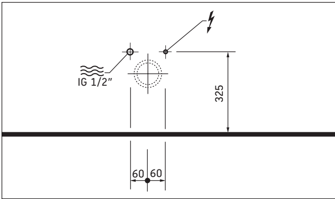
电气连接/水管连接位置
