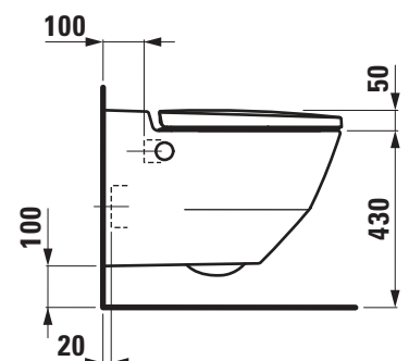
Anschlüsse mit handelsüblichen Installationssystemen
