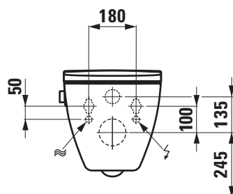
Anschlüsse mit LAUFEN Installationssystem LIS CW2
