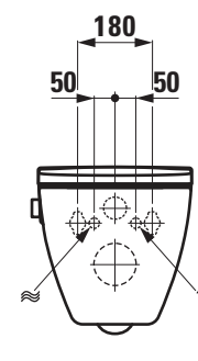
Anschlüsse mit handelsüblichen Installationssystemen
