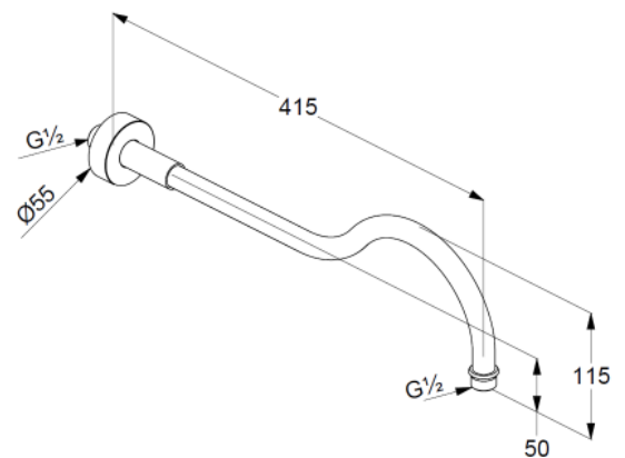
Maßzeichnung/ Dimensional drawing
