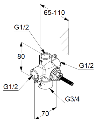
Maßzeichnung
