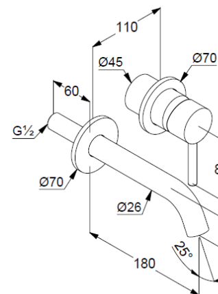
Maßzeichnung/ Dimensional drawing
