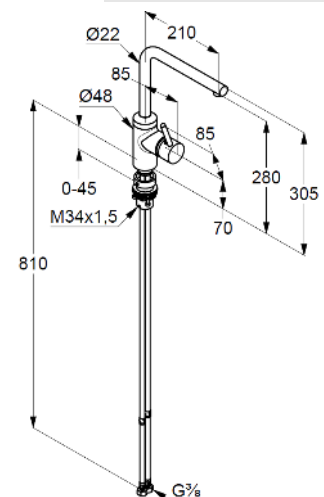
Maßzeichnung
