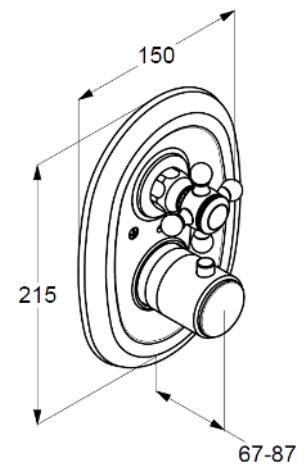
Maßzeichnung/ Dimensional drawing
