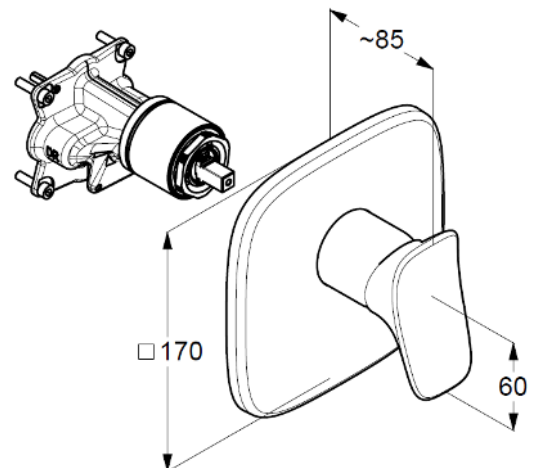
Maßzeichnung
