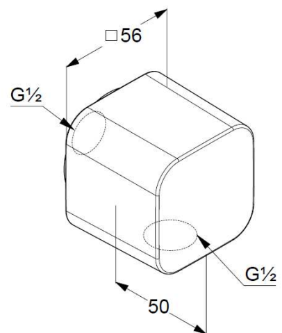
Maßzeichnung
