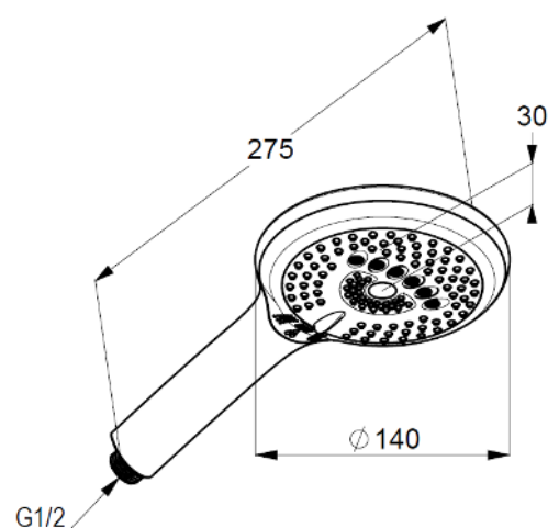
Maßzeichnung
