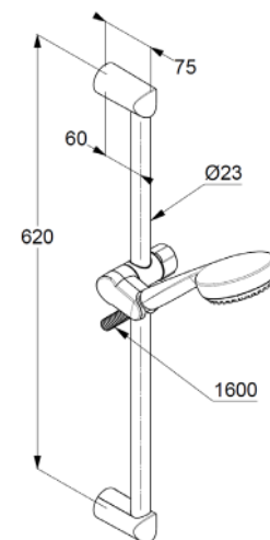
Maßzeichnung/ Dimensional drawing
