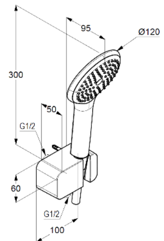
Maßzeichnung
