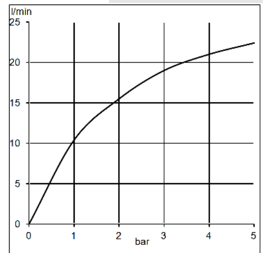
Durchflussdiagramm
