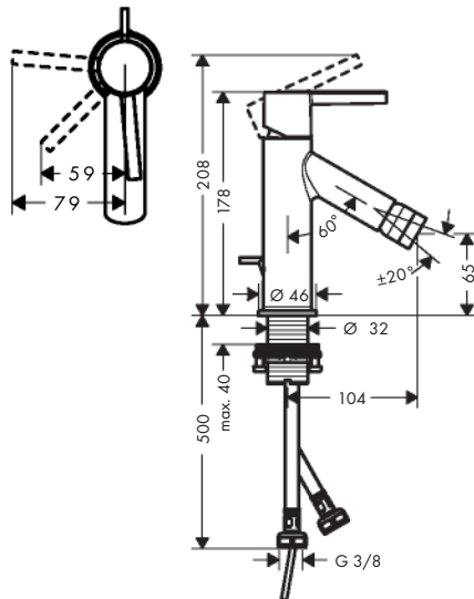
AXOR Starck 10214XXX
