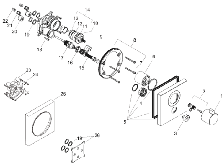
製品分解図
