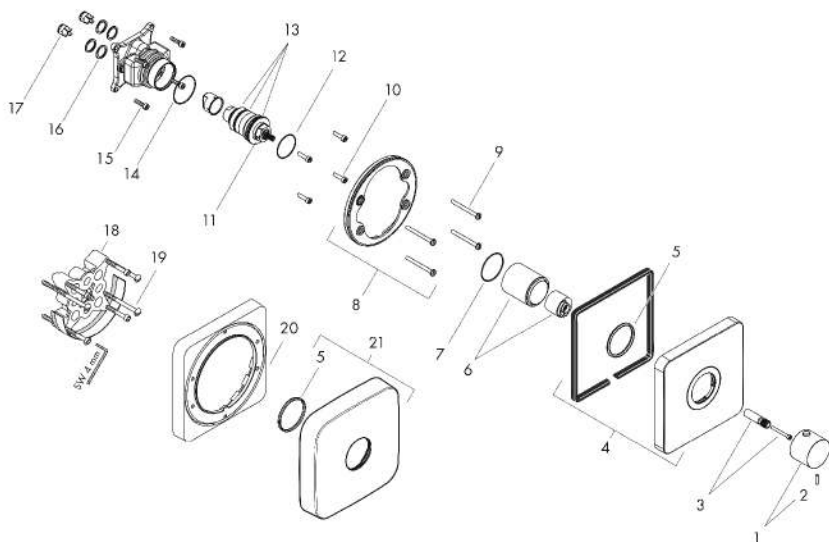
製品分解図
