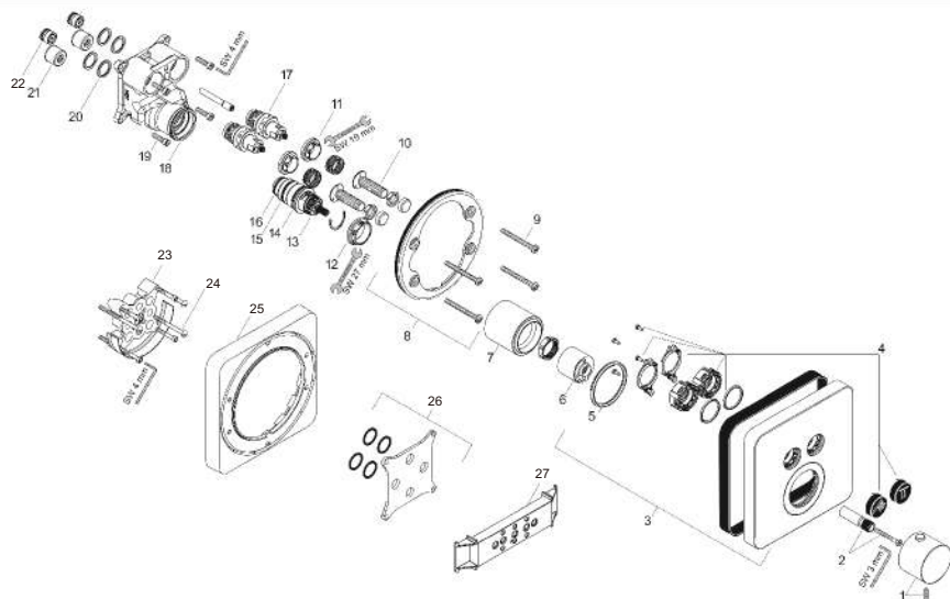
製品分解図
