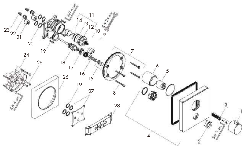
製品分解図
