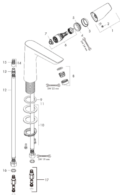
製品分解図
