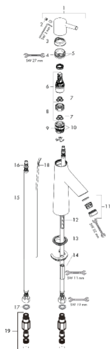
部品リスト
