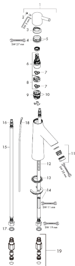
製品分解図
