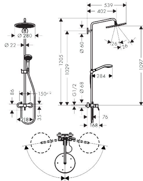
Maßzeichnung
