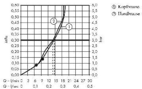
Durchflussdiagramm
