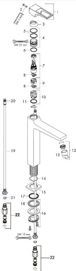
製品分解図
