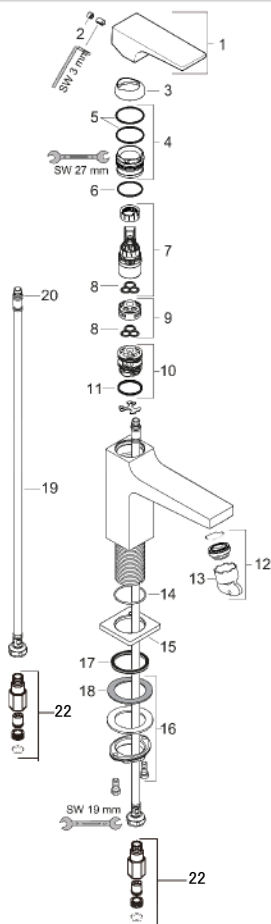
製品分解図
