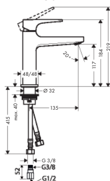
完成図
