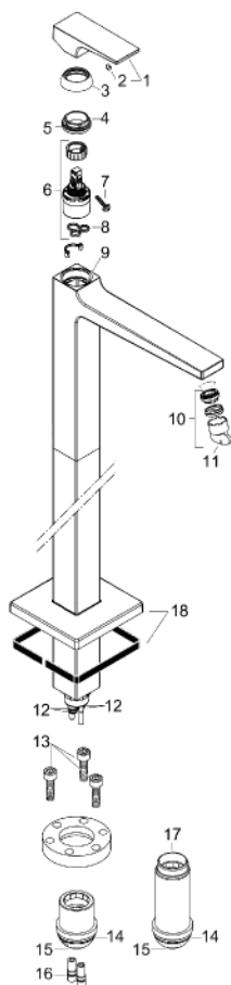
製品分解図
