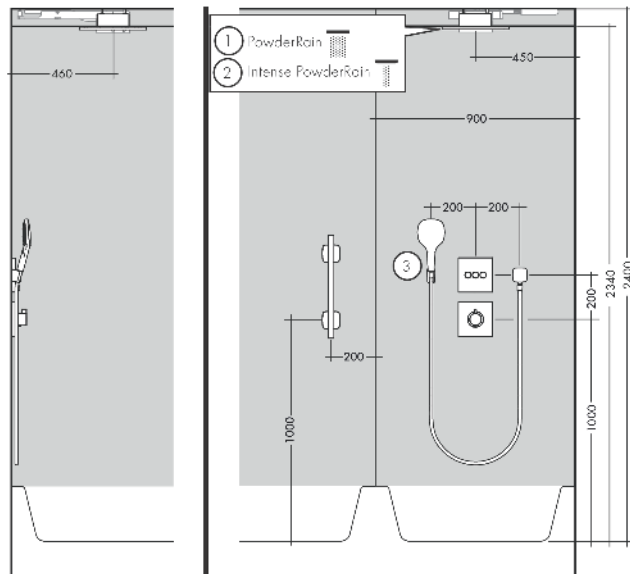
AXOR 250 2jet 35298800 AXOR 300 2jet 35305200
