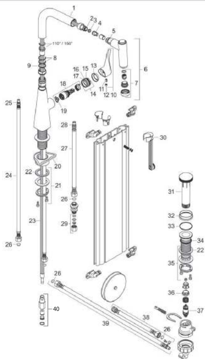
製品分解図
