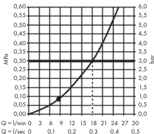
Croma E 280 1jet 26257000
