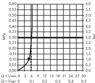
Croma E 280 1jet 26257005
