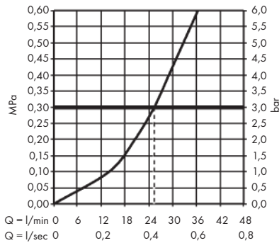
AXOR Edge 46750XX0 / 46751XX0
