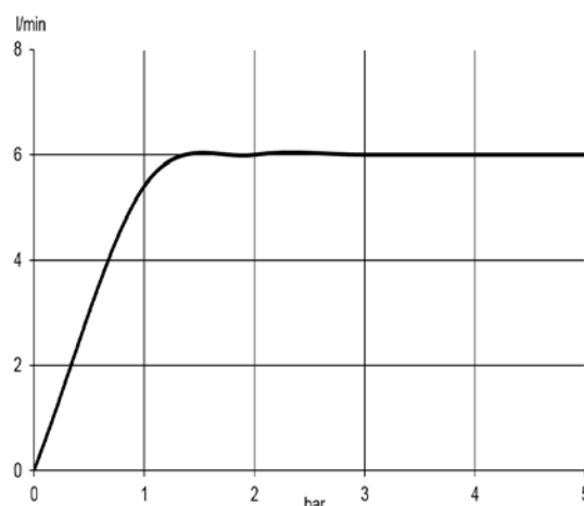
Durchflussdiagramm
