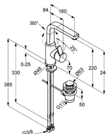
Maßzeichnung
