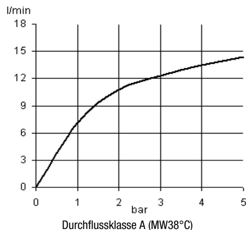
Durchflussdiagramm
