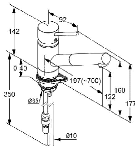
Maßzeichnung
