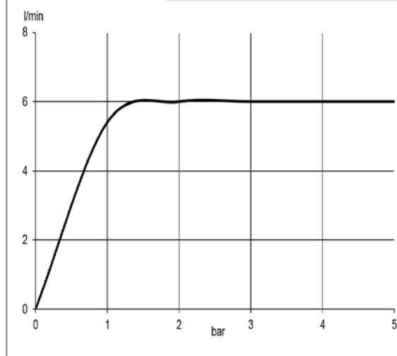
Durchflussdiagramm
