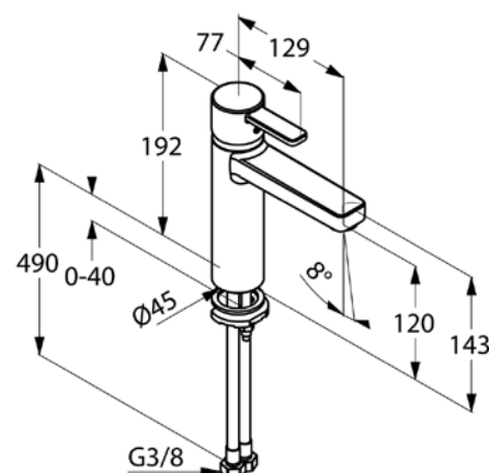
Maßzeichnung
