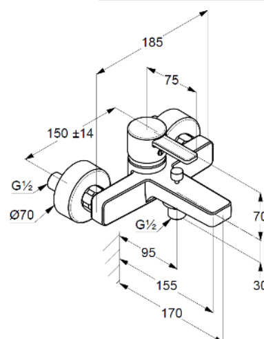
Maßzeichnung
