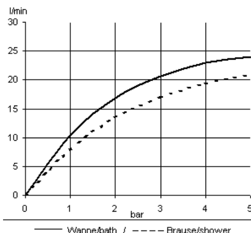
Durchflussdiagramm
